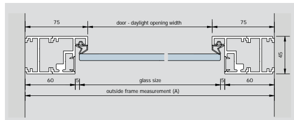
plan / door Type B
