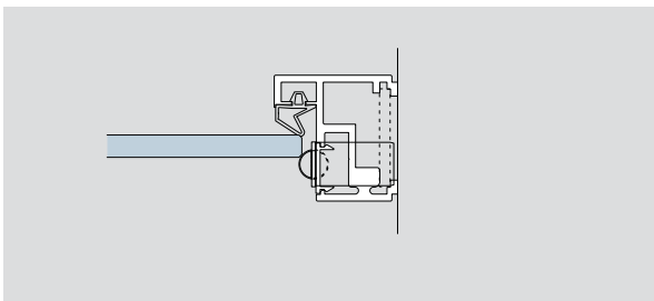
round bolt door catch
