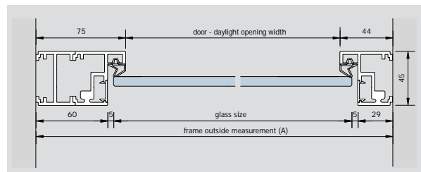
plan / door Type C
