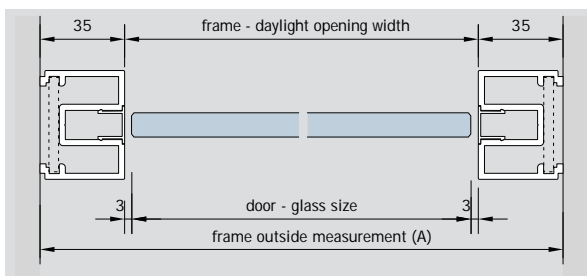
plan / door
